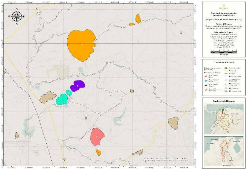
Ilustración 1. Zonas de excedencia del nivel máximo permisible anual de material particulado PM 10 en la zona carbonífera del Cesar.
